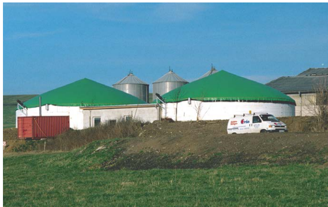
Bild 2: Biogasfermenter mit Foliendach
